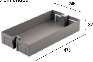
Cesto em chapa
