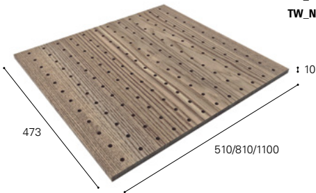
TW_NOG-400 (510) TW_NOG-401 (810) TW_NOG-402 (1100)
