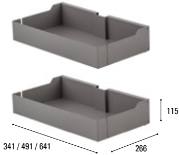
CESTOS INTERIORES Inclui 3 Kits com 2 cestos/cada.
