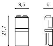
Cabos 0,35~0,75mm 2
