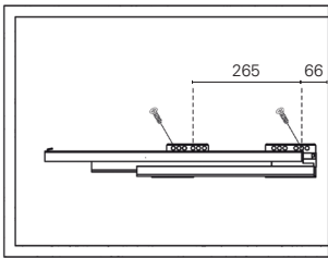
Corrediça oculta de 450mm.
